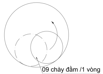
b) Bố trí chày đầm cối nhỏ
