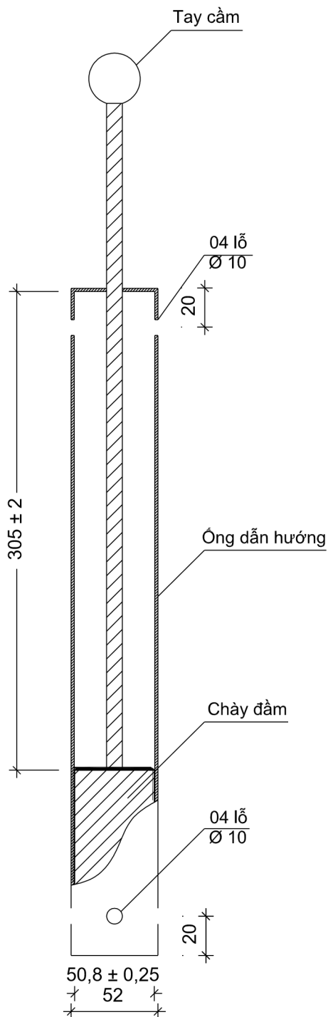
a) Chày đầm
