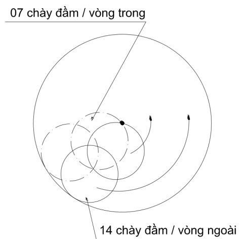
c) Bố trí chày đầm cối lớn
