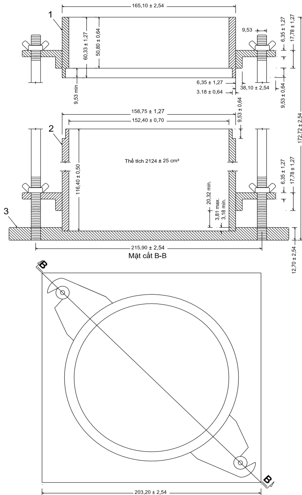
Hình 1 - Cối nhỏ
